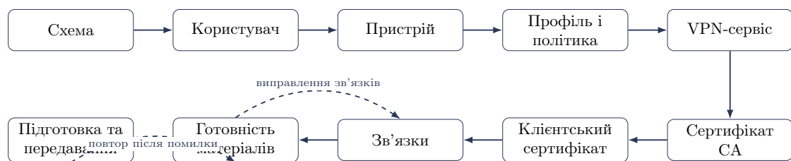
Рис. 2: Поточна станова модель майстра налаштування VPN
