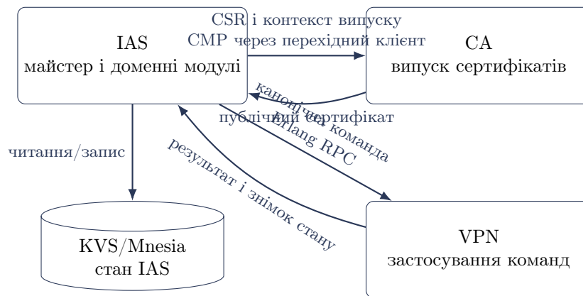
Рис. 3: Архітектурні межі та взаємодія IAS, CA, VPN і KVS/Mnesia
