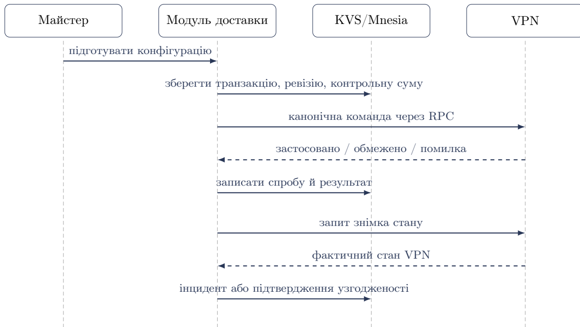
Рис. 4: Послідовність передавання конфігурації та звіряння стану
