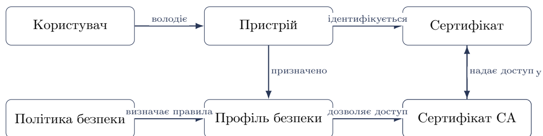
Рис. 1: Поточна доменна модель IAS та основні зв'язки
