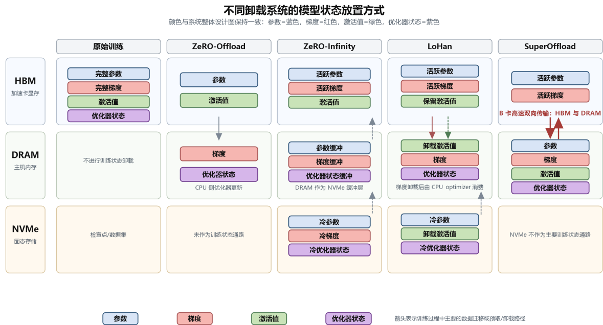
图 2.3 不同卸载系统中模型状态在 HBM、DRAM 与 NVMe 间的放置方式
