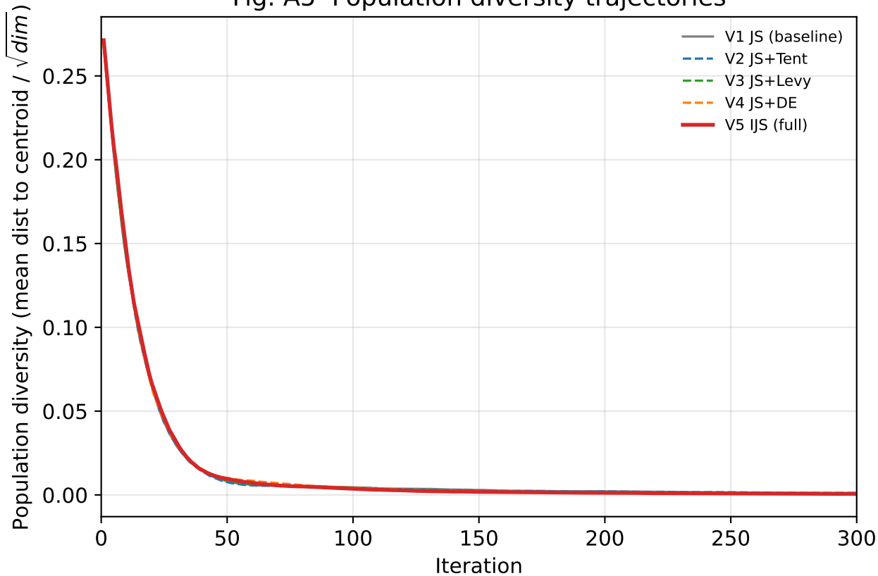
Fig. A5 Population diversity trajectories
