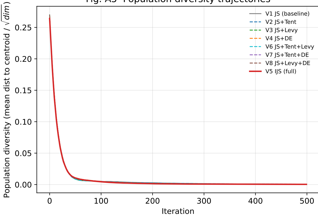
Fig. A5 Population diversity trajectories
