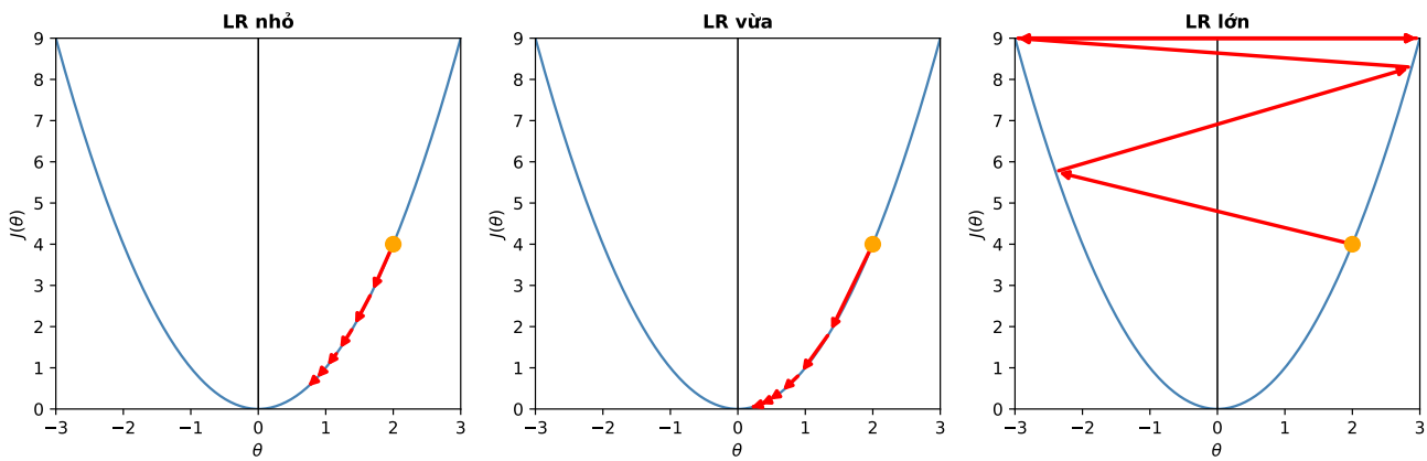
Hình 16: Ảnh hưởng của learning rate ( \eta ) đến quá trình hội tụ của Gradient Descent. Bên trái: \eta nhỏ dẫn đến hội tụ chậm. Giữa: \eta vừa phải giúp hội tụ hiệu quả. Phải: \eta lớn dẫn đến dao động và không thể hội tụ.
