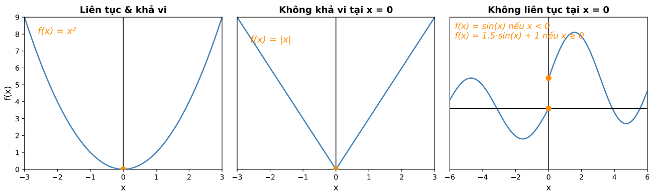
Hình 17: Minh họa các loại hàm mục tiêu. Từ trái qua: Hàm liên tục và khả vi, hàm không khả vi tại x=0 , và hàm không liên tục tại x=0 .
