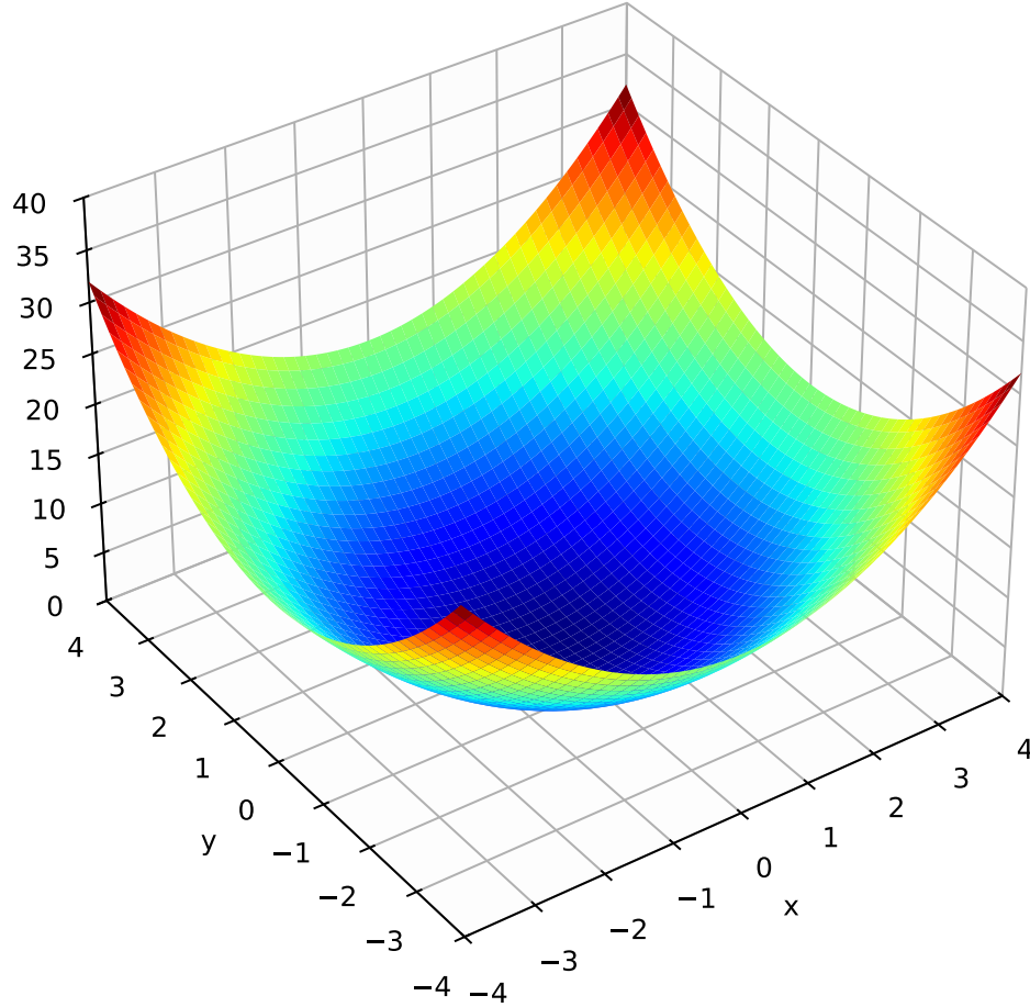
Hình 14: Hàm f(x, y) = x^2 + y^2 . Màu sắc thể hiện độ cao của bề mặt. Quỹ đạo di chuyển của Gradient Descent được mô tả như quá trình “trượt xuống” đáy parabol.
