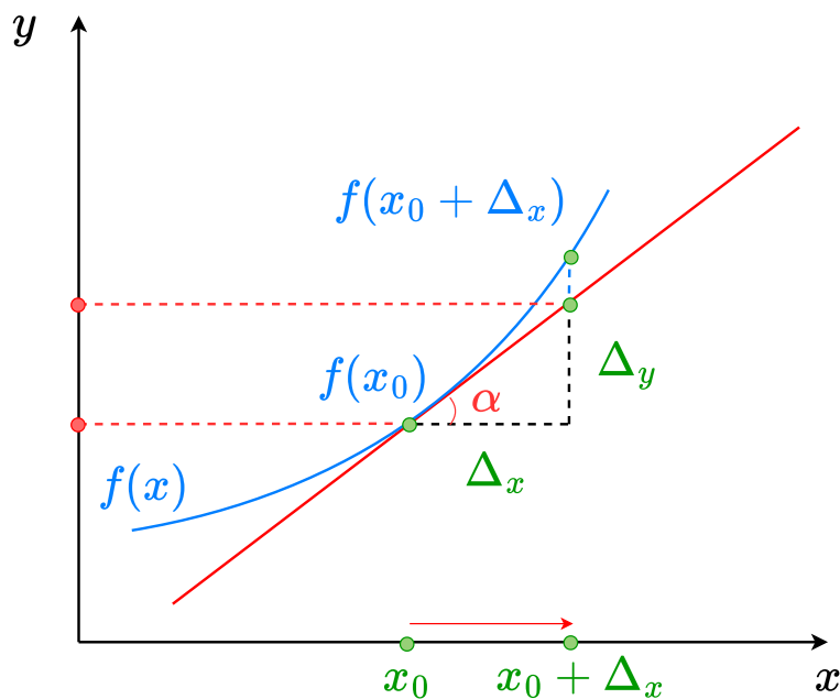
Hình 5: Mô tả đạo hàm của hàm số y = f(x) sau khi x thay đổi một đoạn \Delta x .
