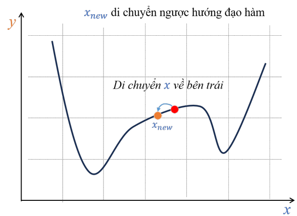
(b) Áp dụng tính chất đi ngược hướng đạo hàm để tiến về cực tiểu.
