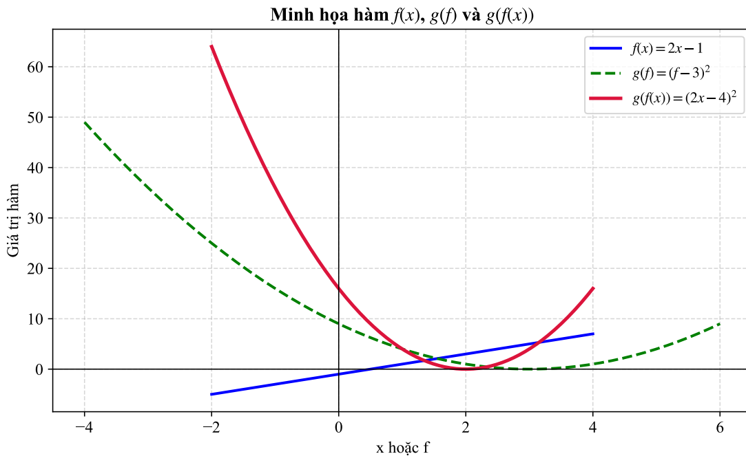
Hình 15: Minh họa hàm f(x) = 2x - 1 , g(f) = (f - 3)^2 và hàm hợp g(f(x)) = (2x - 4)^2 . Đường đỏ cho thấy hình dạng tổng thể của hàm hợp cần tối ưu.
