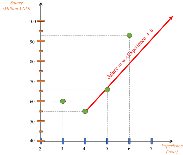
Hình 2: Minh họa một đường thẳng tuyến tính trên trục tọa độ.
