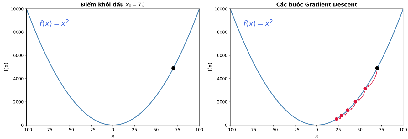
Hình 13: Quá trình Gradient Descent trên hàm f(x) = x^2 . Các mũi tên biểu diễn hướng di chuyển ngược chiều đạo hàm từ điểm khởi tạo x_0 = 70 về điểm cực tiểu toàn cục x = 0 .
