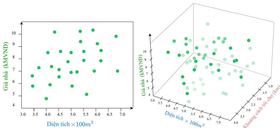
Hình 2: Các điểm dữ liệu rời rạc trong không gian 2D và 3D.
