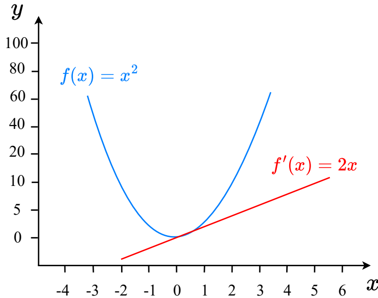
Hình 8: Minh họa cho ví dụ về tính toán phương trình đạo hàm.
