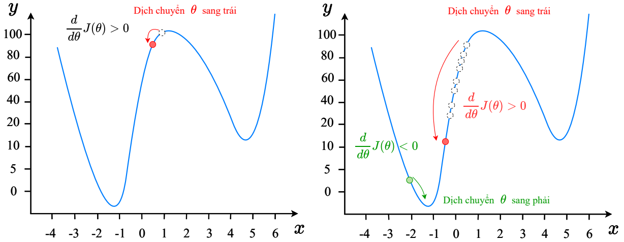
Hình 11: Đi ngược hướng đạo hàm để tiến về giá trị tối ưu \theta_{opt} .
