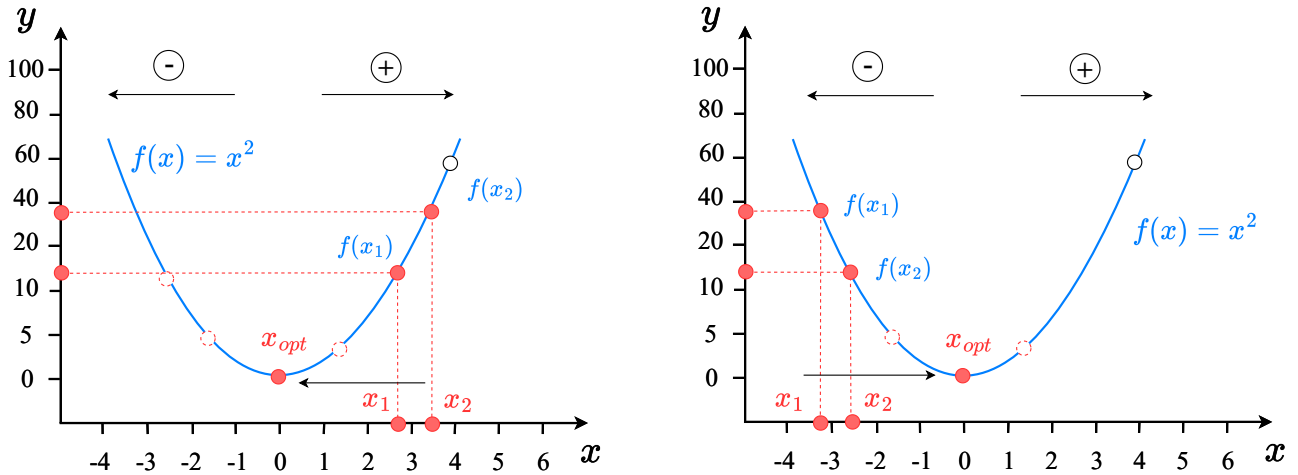
Hình 10: Minh họa cho chiều giá trị của đạo hàm khi ta thay đổi giá trị của x .
