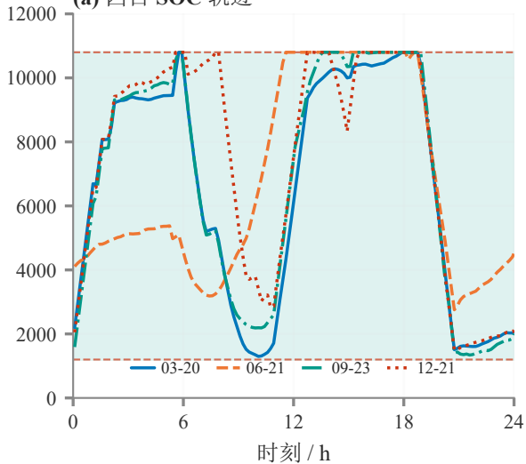
(a) 四日 SOC 轨迹
