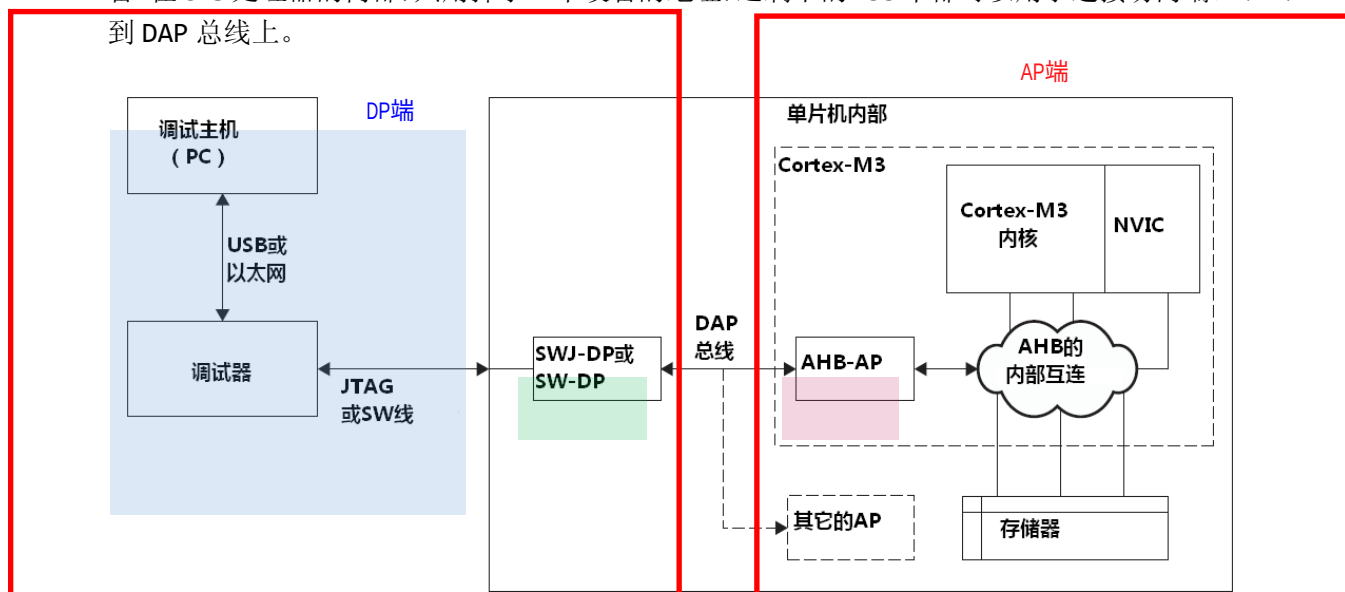
图 15.1 高度主机到 Cortex-M3 的连接
