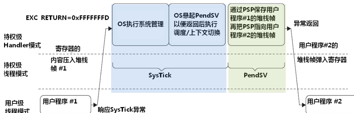
图 12.3 SysTick 异常推动简单轮转调度模式图
