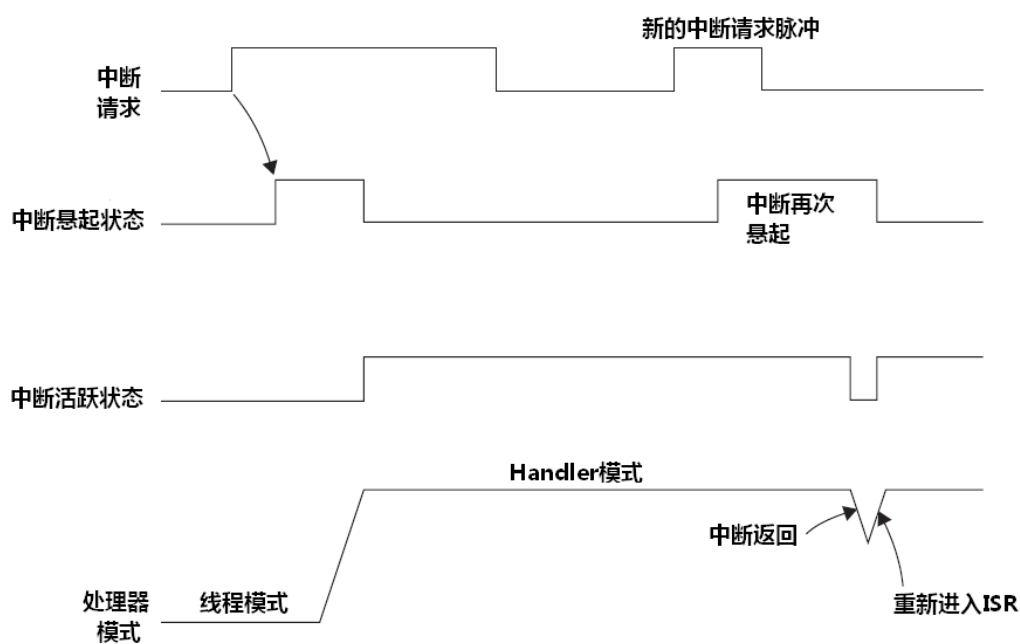
图 7.13 在执行 ISR 时中断悬起再次发生
