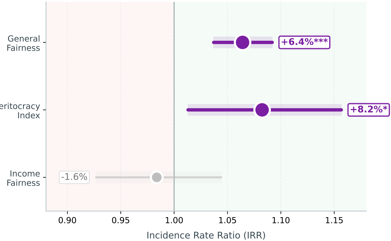
Poisson Regression
