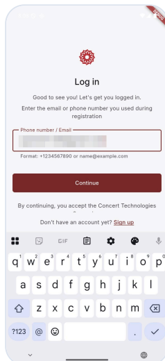
02 · Authentication – login-filled
