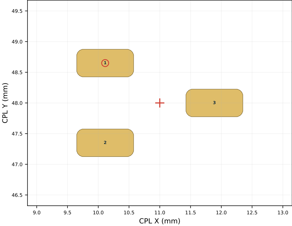
U4 | anchor (11.0000, 48.0000) mm | 0° top
