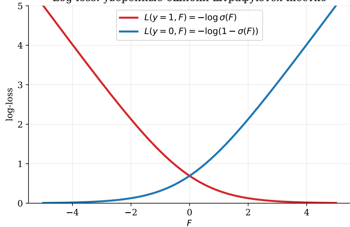
Log-loss: уверенные ошибки штрафуются жёстко
