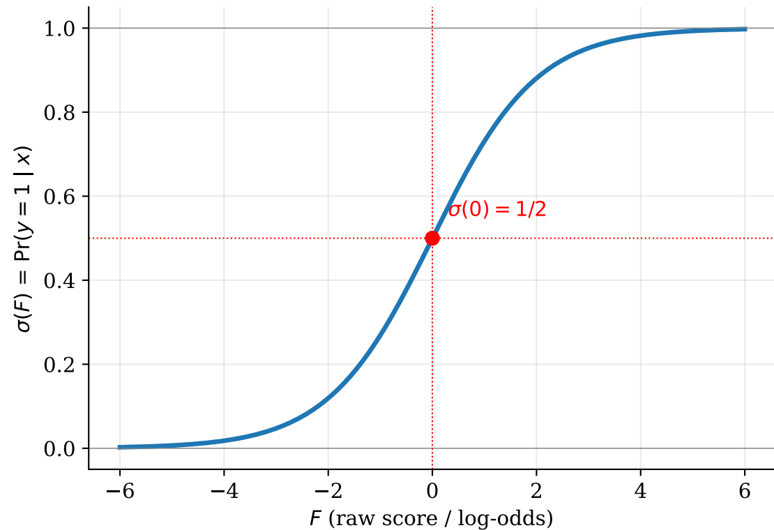
Сигмоида: \mathbb{R} \rightarrow [0, 1]
