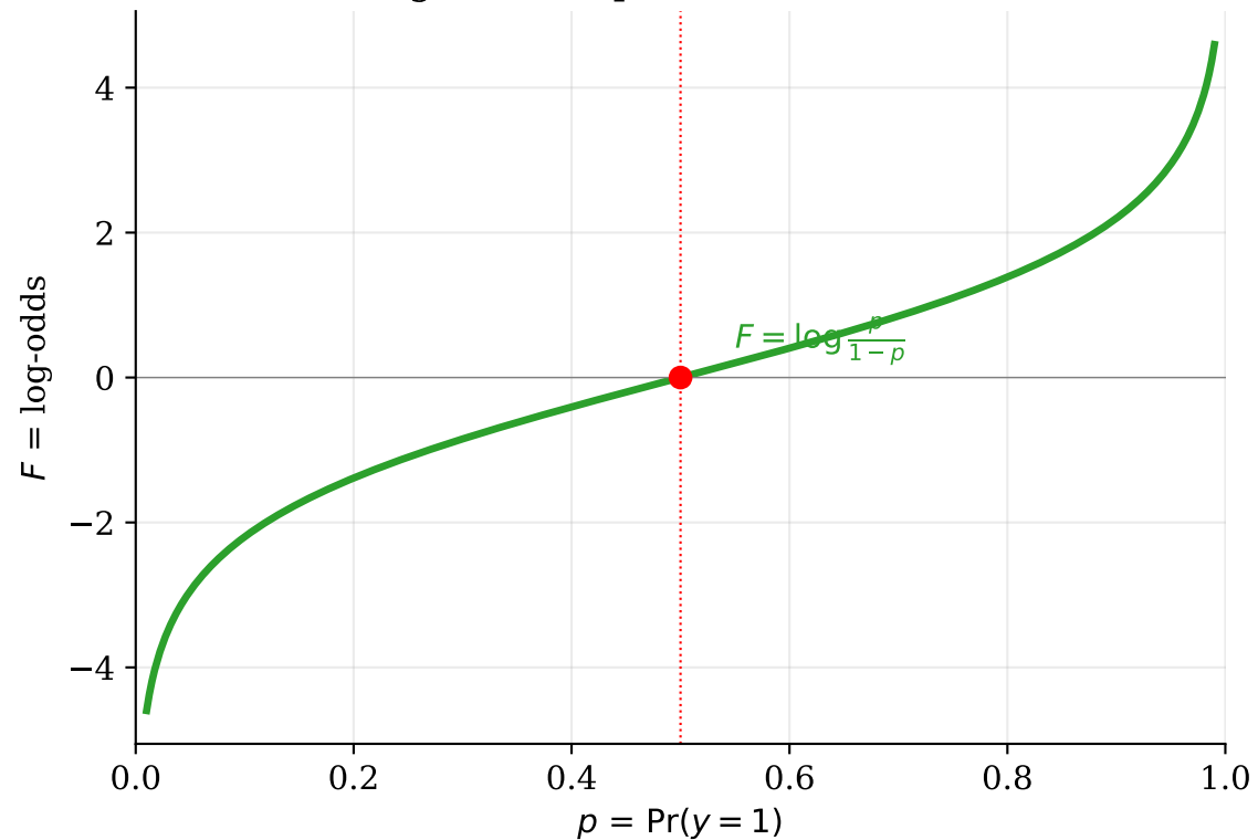
Log-odds: обратная к сигмоиде
