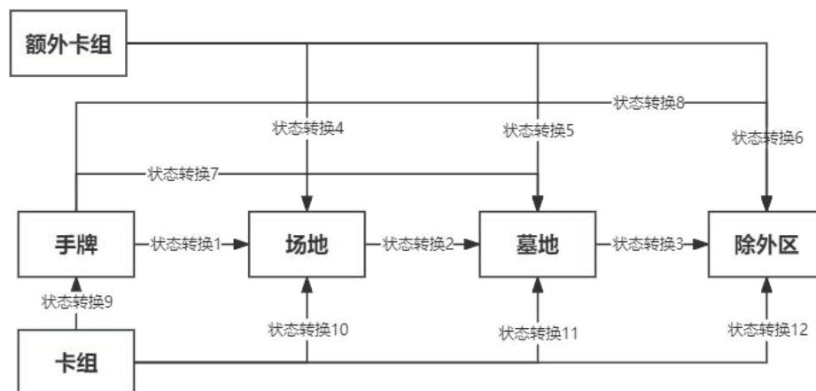
卡牌状态转换流程图
