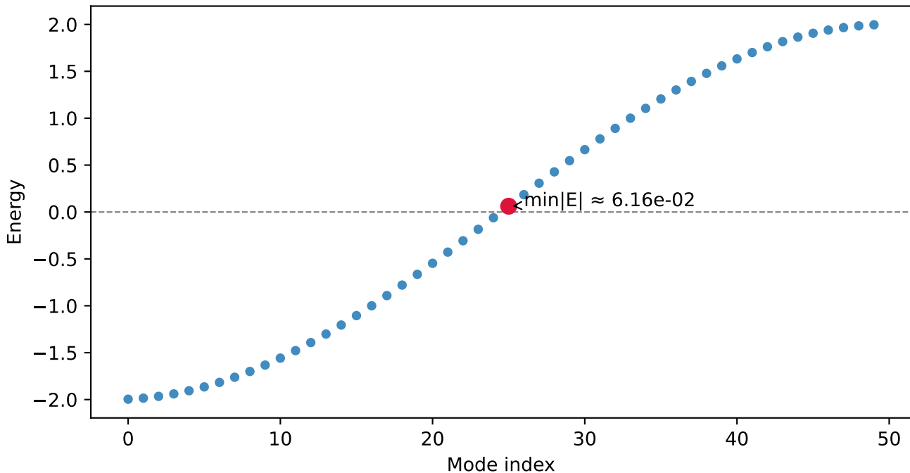
SSH Spectrum ( N=50 , \lambda=0.0 , OBC)
