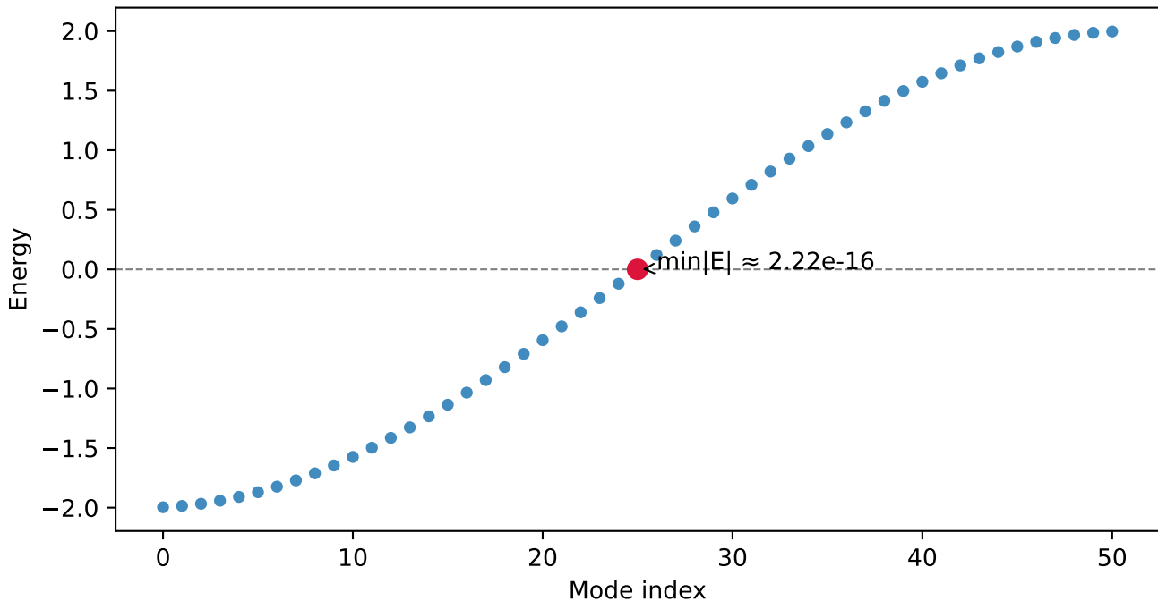
SSH Spectrum ( N=51 , \lambda=0.0 , OBC)
