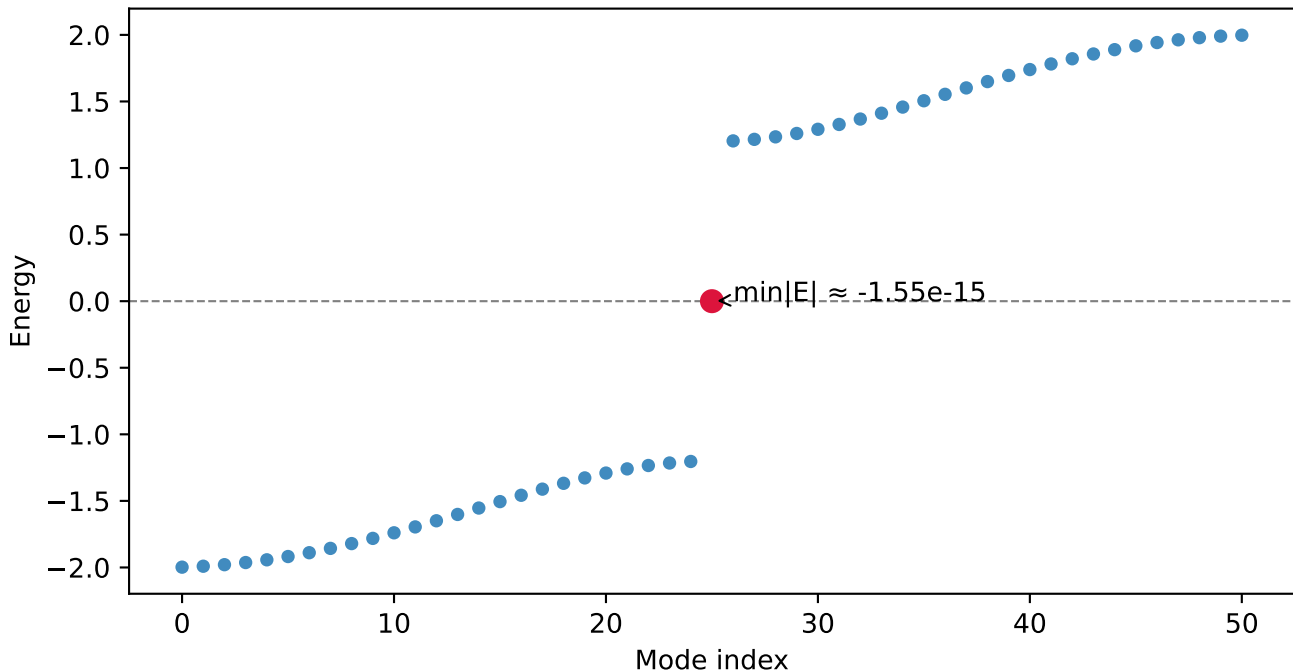
SSH Spectrum ( N=51 , \lambda=0.6 , OBC)
