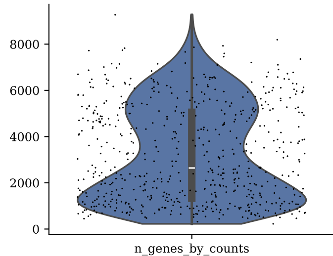
Genes per spot
