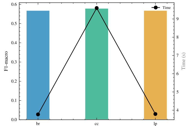
(B) F1 vs Time Cost (PML)
