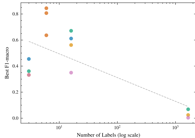
(D) Label Complexity vs F1 ( r=-0.71 )
