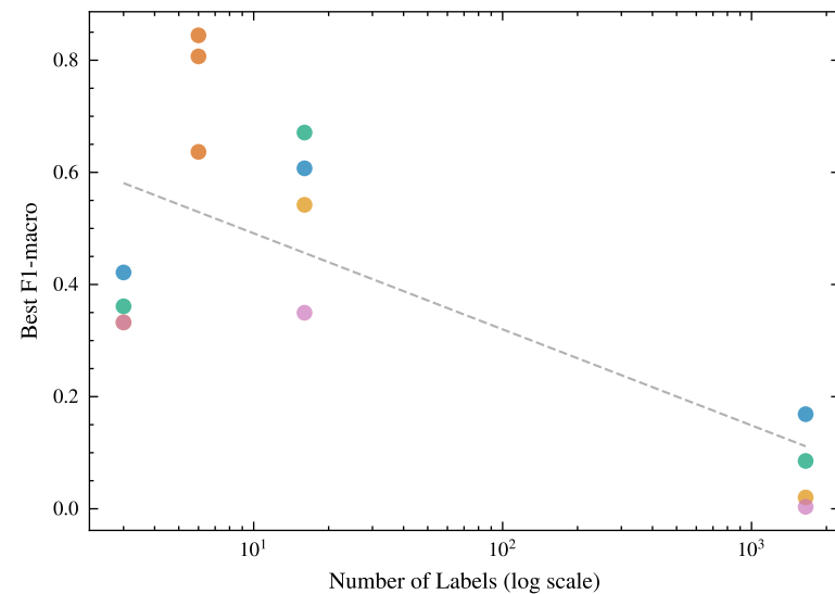
(D) Label Complexity vs F1 ( r=-0.72 )
