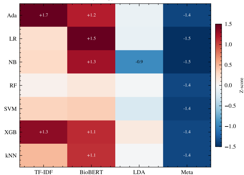
(D) Feature × Model Synergy (Z-score)
