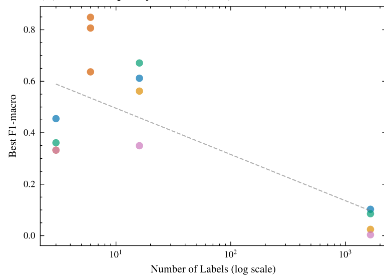
(D) Label Complexity vs F1 ( r=-0.74 )
