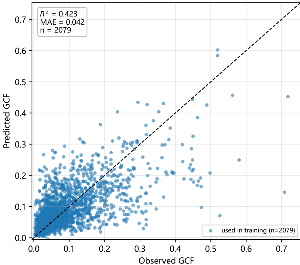
GCF — Holdout_B0CV
