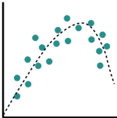
恰当的拟合
