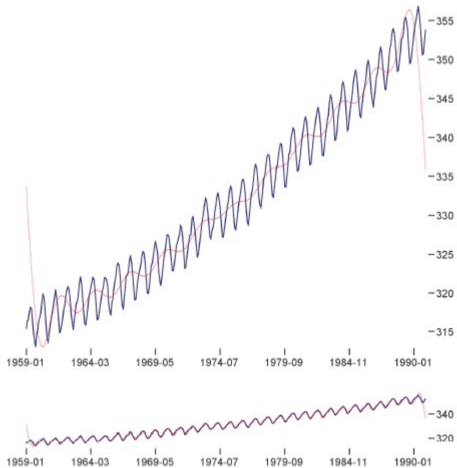
二氧化碳浓度变化
