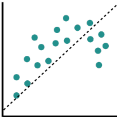
欠拟合
