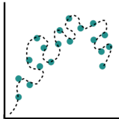
过拟合
