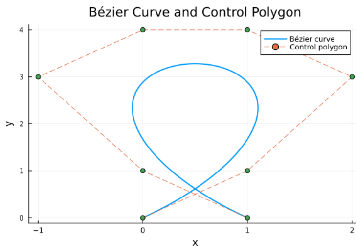
Slika 1: Bézierjeva krivulja, ki je predmet te naloge.
