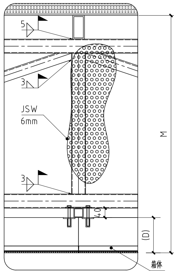
显示屏"平面-中"节点大样图
