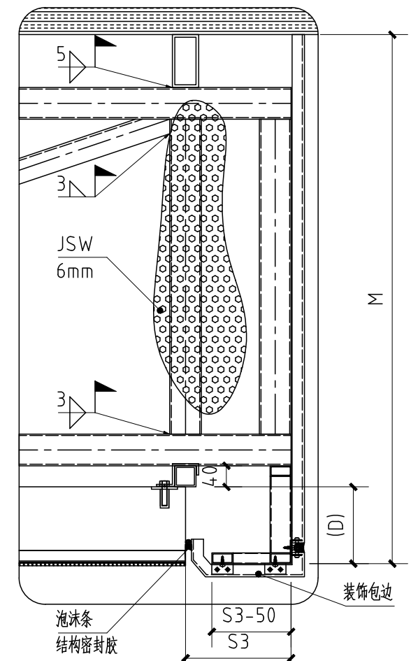
显示屏"平面-侧"节点大样图
