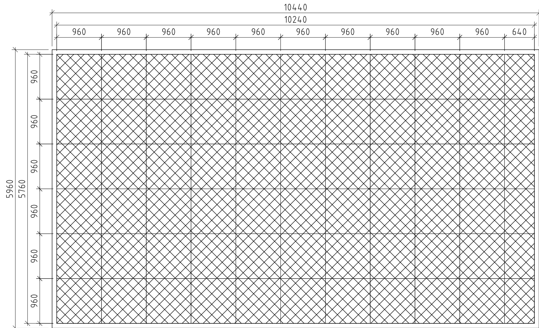
显示屏正立面图
