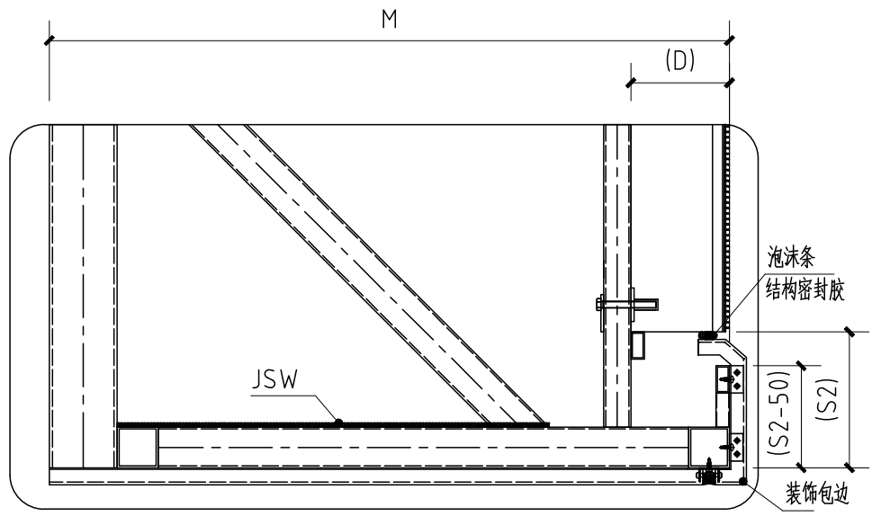
显示屏底部侧剖节点大样图
