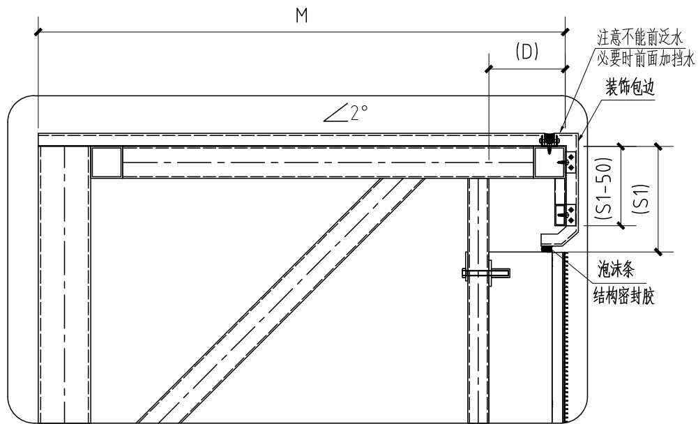
显示屏顶部侧剖节点大样图
