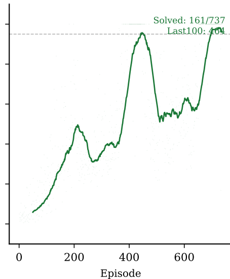
A2C
