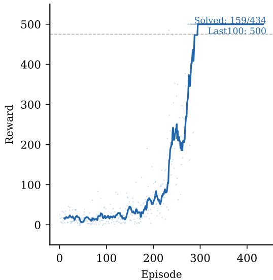
PPO
