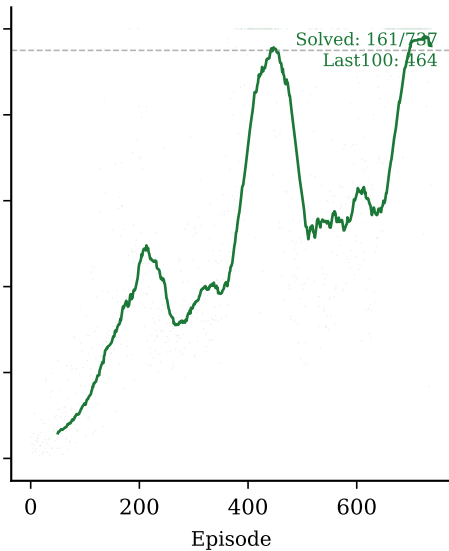
A2C
