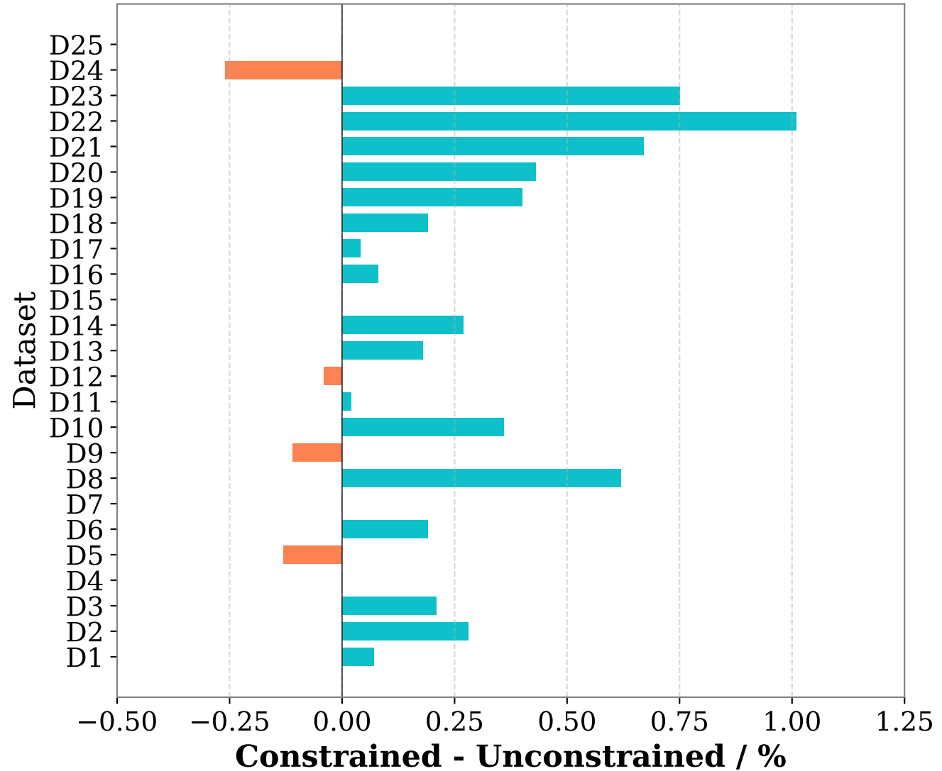
AUC
