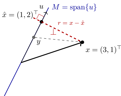
图 1.3: x = (3, 1)^T 到直线 M = \text{span}\{(1, 2)^T\} 的正交投影：垂线段 x\hat{x} 最短，而 M 上任何其他点 y 满足 \|x - y\|_2 > \|x - \hat{x}\|_2
