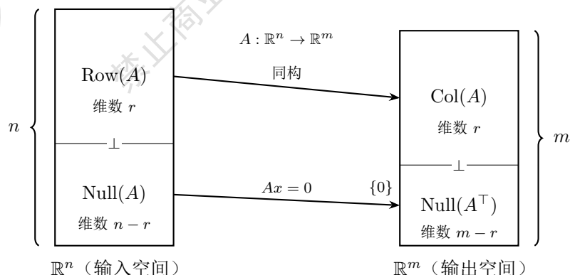
图 1.2: 矩阵 A \in \mathbb{R}^{m \times n} 的四个基本子空间及其维数 ( r = \text{rank}(A) )
