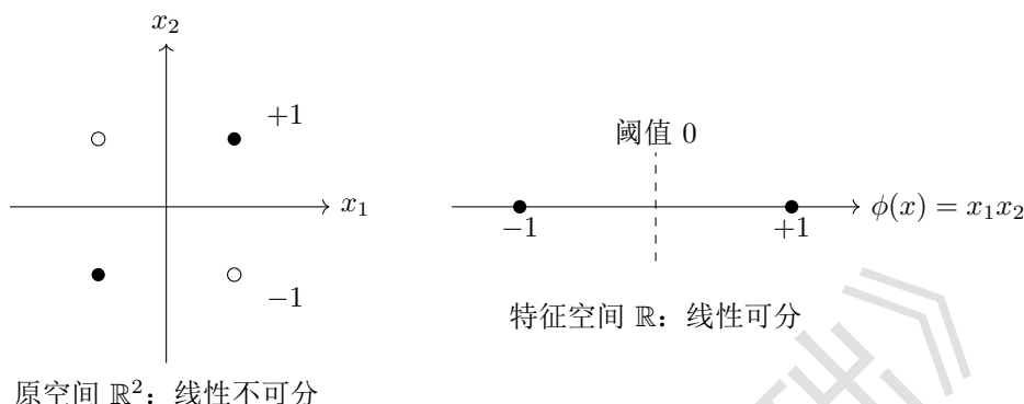
图 1.6: XOR 问题：特征映射 \phi(x_1, x_2) = x_1x_2 把线性不可分变为线性可分
