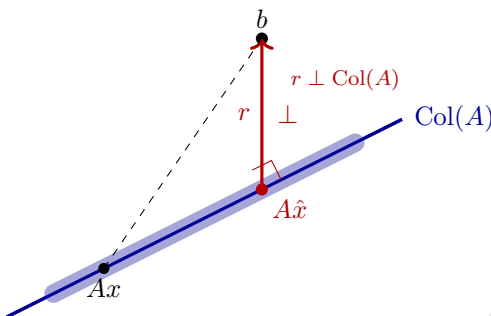
图 1.4: 最小二乘的几何解释: 在 \text{Col}(A) 中寻找距 b 最近的点, 即正交投影 A\hat{x} ; 残差 r = b - A\hat{x} 垂直于 \text{Col}(A) , 而 \text{Col}(A) 中任何其他点 (如 Ax ) 到 b 的距离都更长
