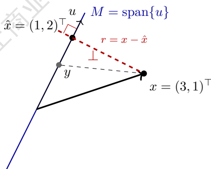
图 1.3: x = (3, 1)^\top 到直线 M = \text{span}\{(1, 2)^\top\} 的正交投影: 垂线段 x\hat{x} 最短, 而 M 上任何其他点 y 满足 \|x - y\|_2 > \|x - \hat{x}\|_2
