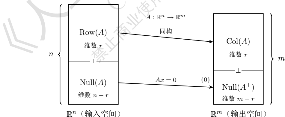
图 1.2: 矩阵 A \in \mathbb{R}^{m \times n} 的四个基本子空间及其维数 ( r = \text{rank}(A) )
