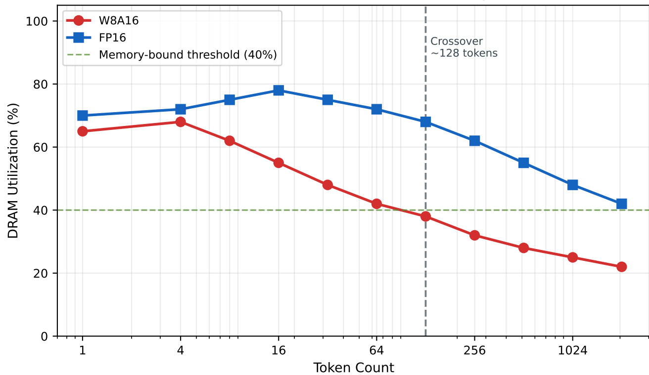
(D) DRAM Bandwidth Utilization (kernel-compass)
