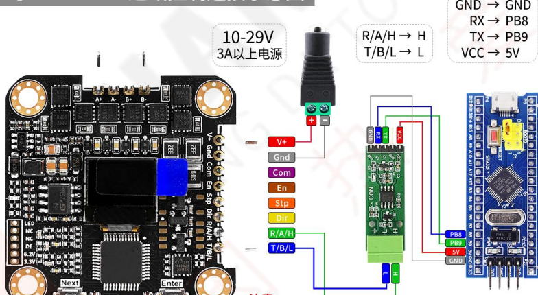
与STM32CAN通讯控制连接示意图
