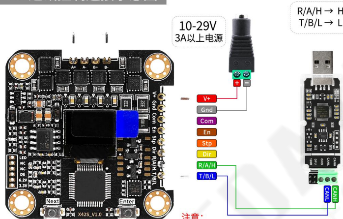
与CAN通讯控制连接示意图
