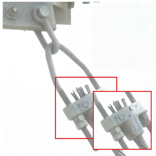
33.57 dB
