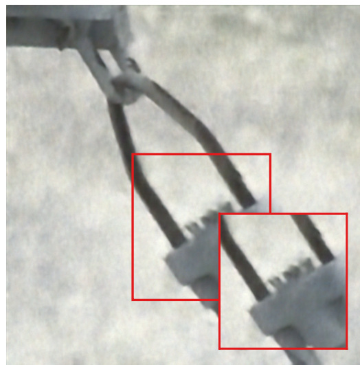
PromptIR 21.31 dB
