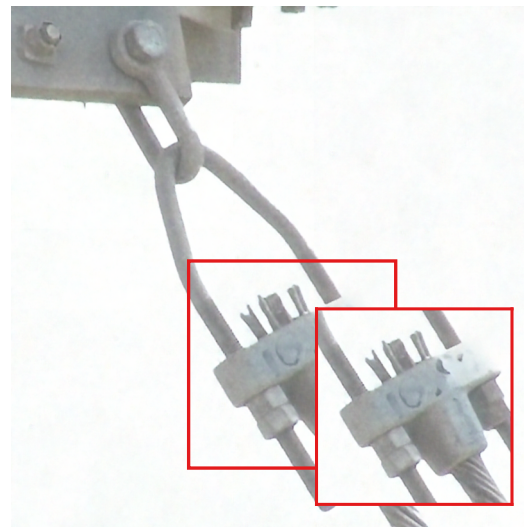
35.83 dB
