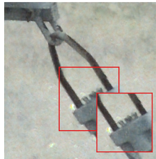
Ours 29.87 dB
