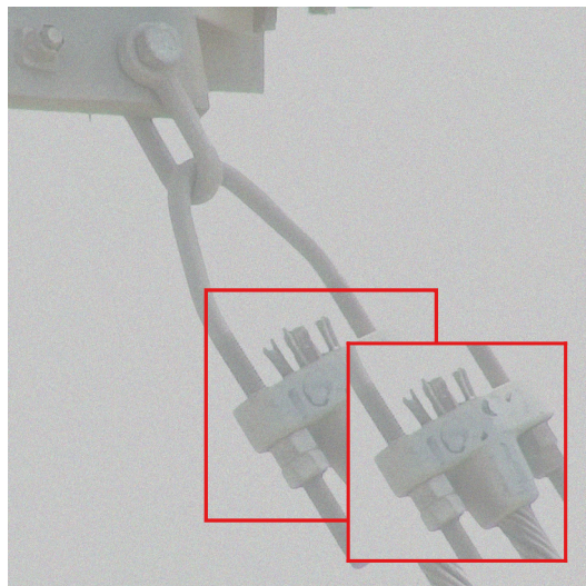
14.33 dB
