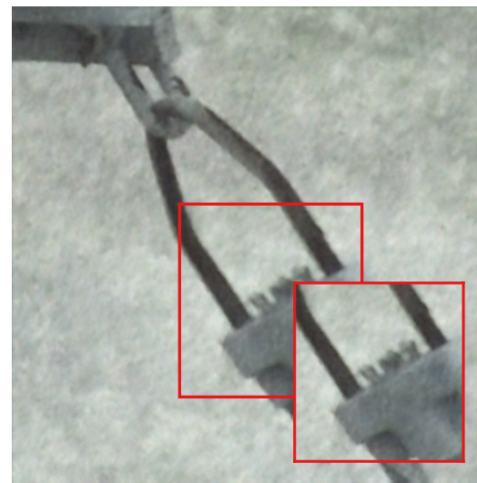
DFPIR 28.64 dB
