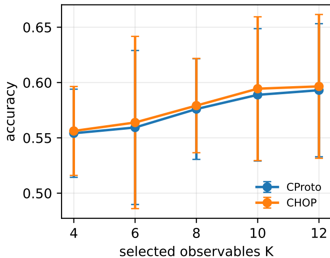
Qiskit Aer MNIST-4
