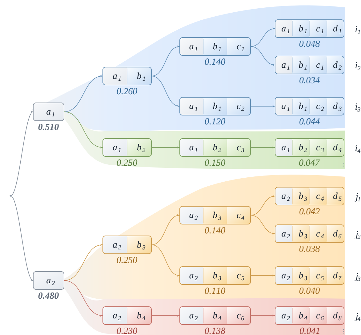
SID layer 1 SID layer 2 SID layer 3 SID layer 4
