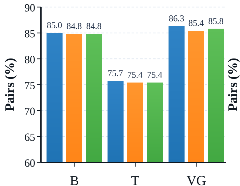
Mixed-sign pairs
