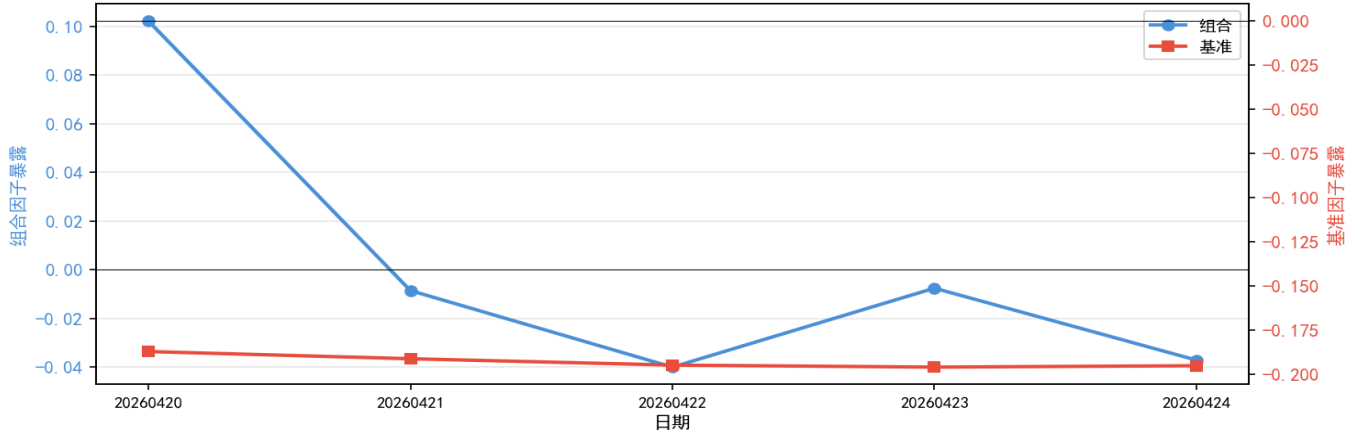
残差波动 因子敞口
