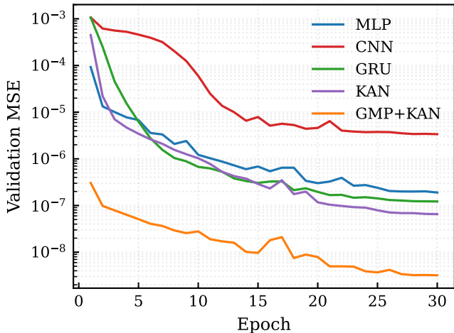
Validation MSE convergence — rapp
