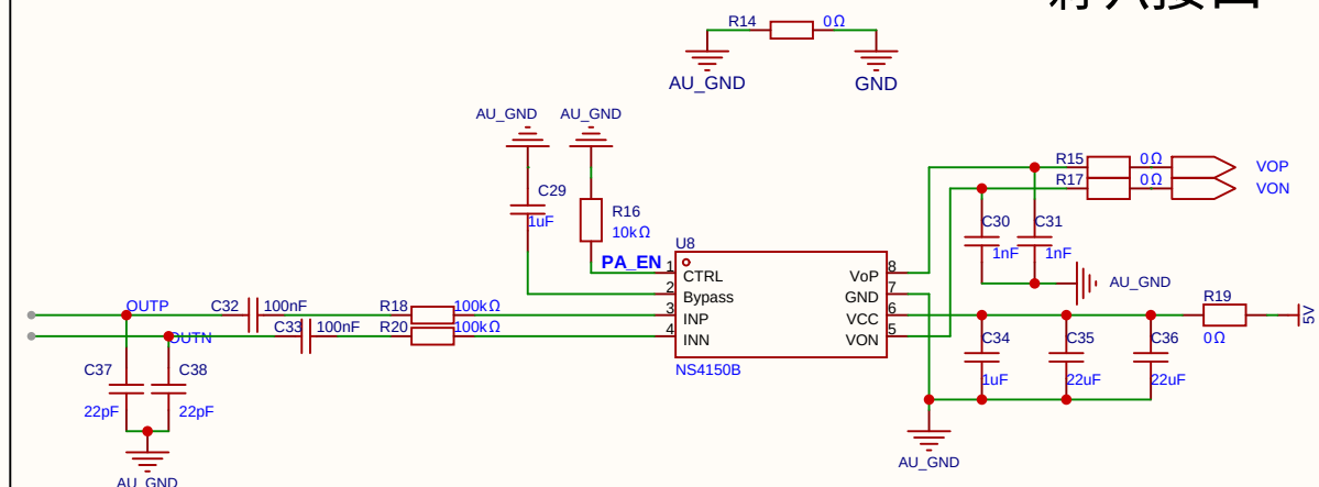
喇叭接口
