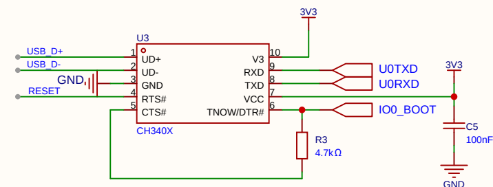
自动下载电路
