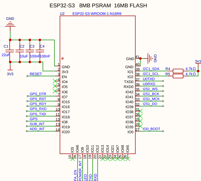
主控MCU
