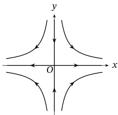
(c) 鞍点
