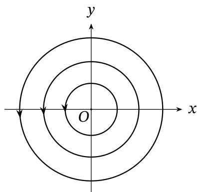
(f) 中心
