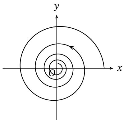
(e) 焦点
