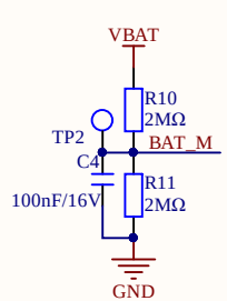
电池电压检测
