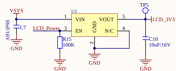
屏幕供电
