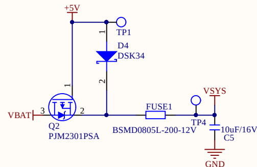
电源选择
