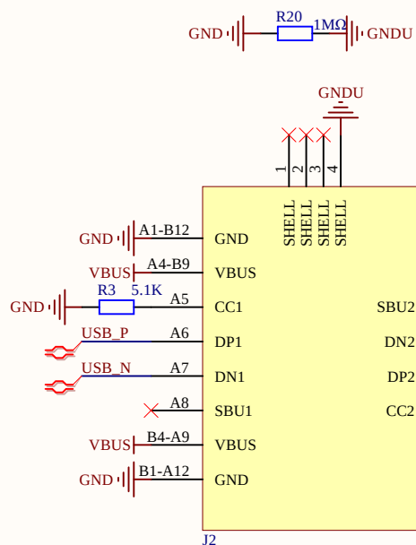
Type-C接口
