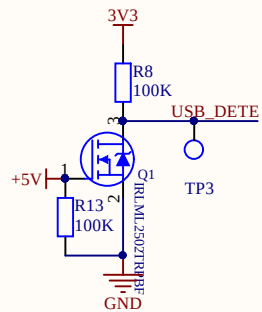
USB检测
