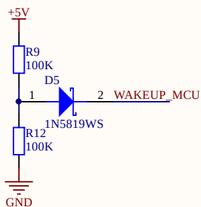
USB唤醒
