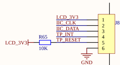
触摸屏接口
