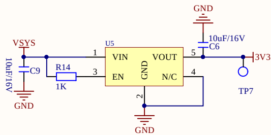
MCU供电
