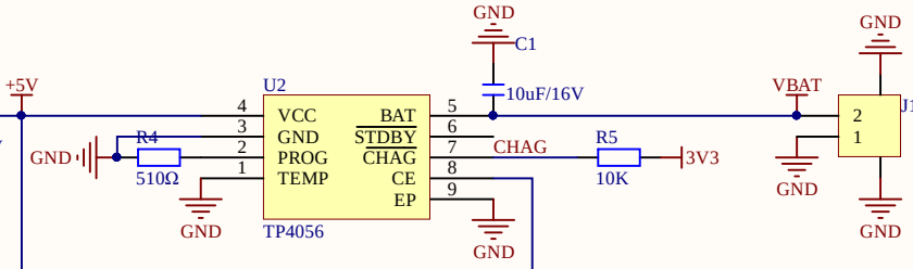
锂电池充电管理
