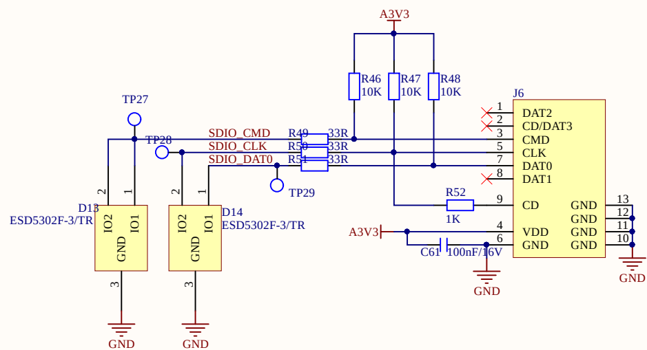
SD卡座
