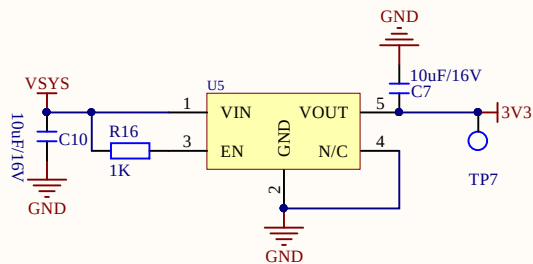
MCU供电
