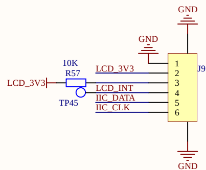
触摸屏接口
