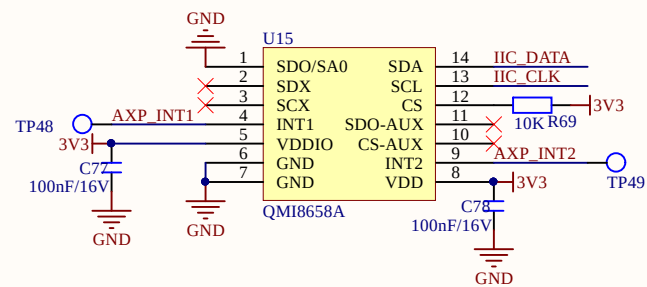
陀螺仪
