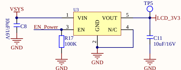
屏幕供电
