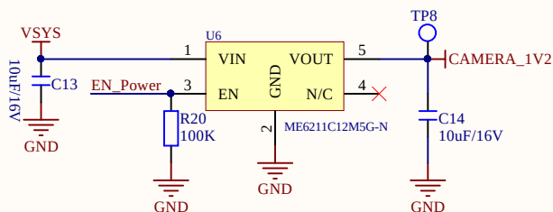
摄像头内核供电
