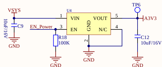
音频芯片/摄像头供电
