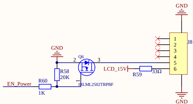
背光接口
