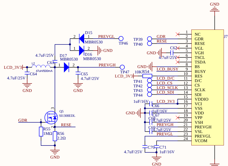
屏幕接口
