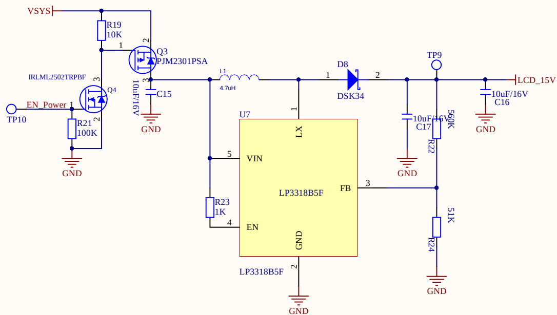
屏幕背光供电
