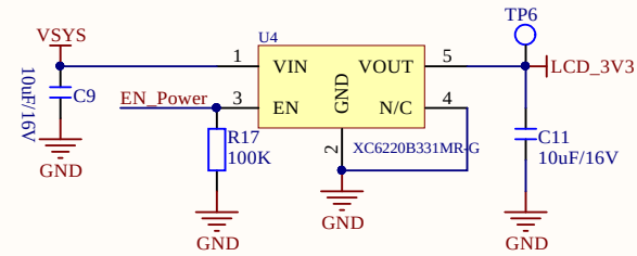
LCD屏幕供电
