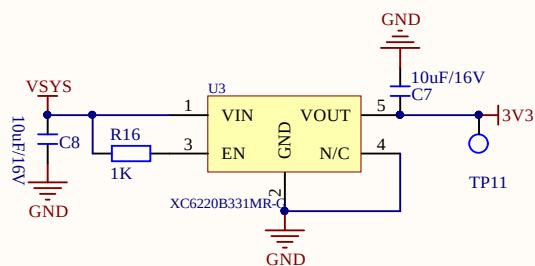
MCU供电
