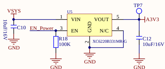
音频芯片供电
