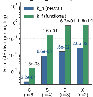
B k_n / k_f decomposition
