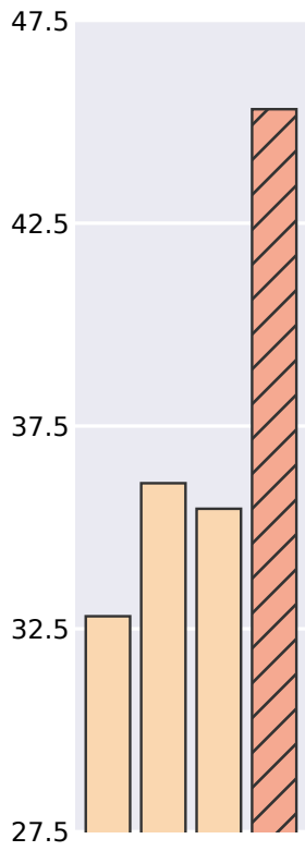
AMC23
