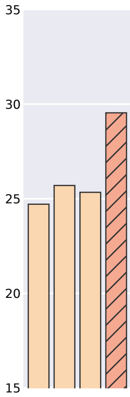
Minerva Math
