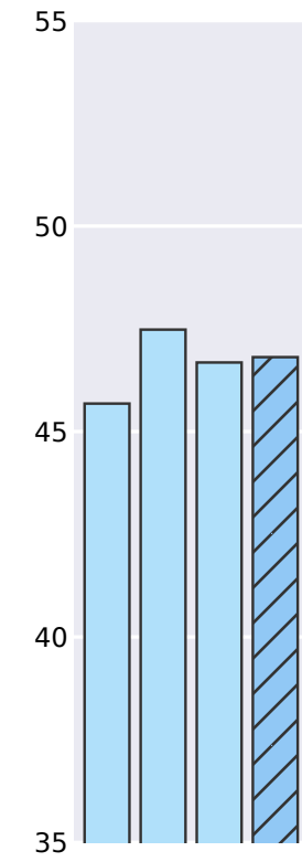
MMLU
