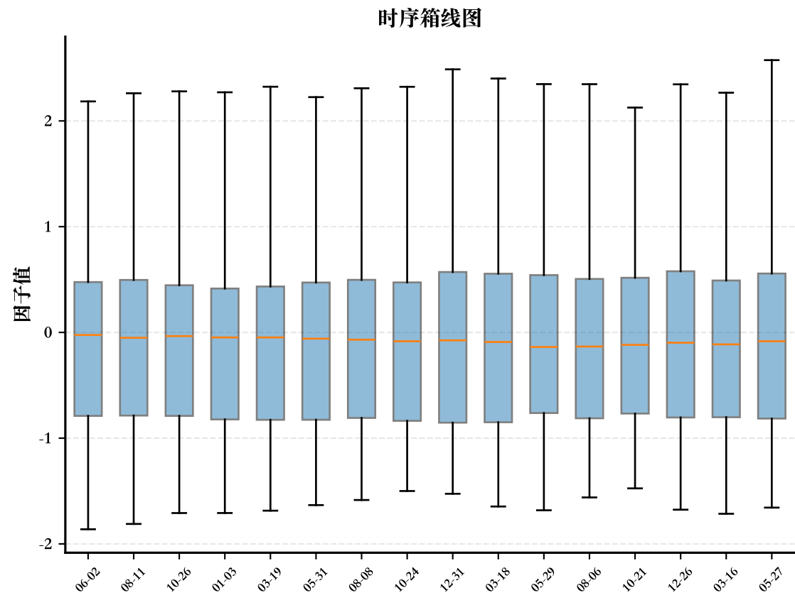
因子分布: size_z
